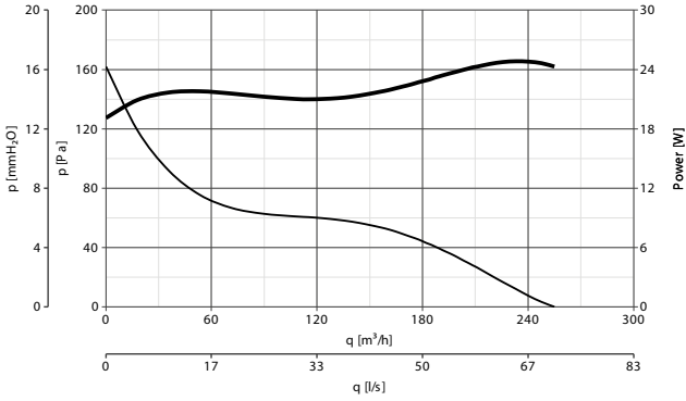
LINEO 100 T - VELOCITÀ MAX
