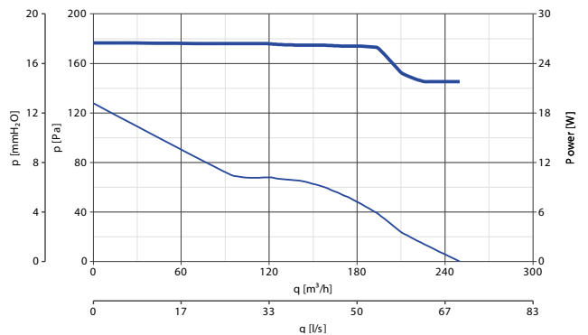
LINEO 125 - LINEO 125 T - VELOCITÀ MIN
