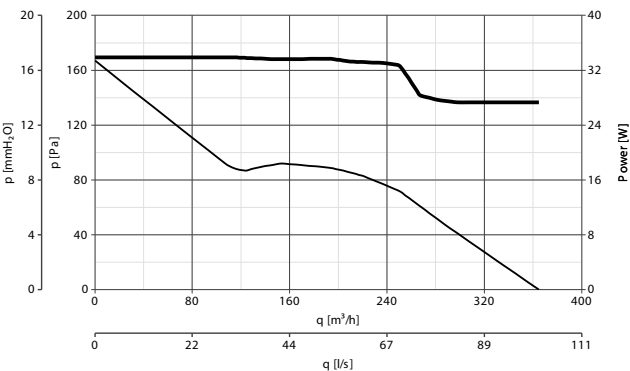
LINEO 125 - LINEO 125 T - MVELOCITÀ MAX
