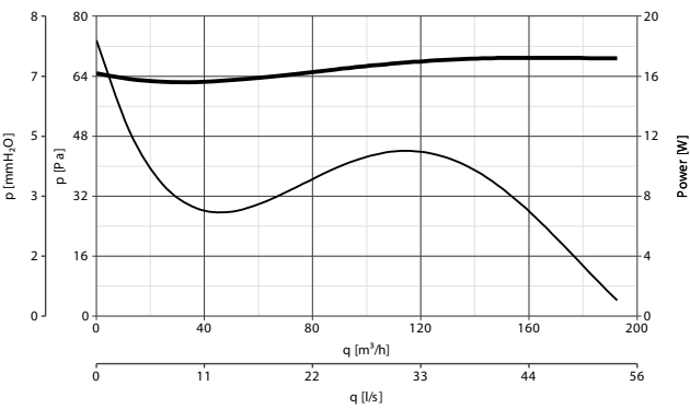
LINEO 100 Q - LINEO 100 Q T - VELOCITÀ MAX
