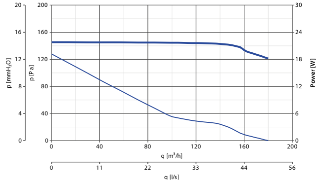
LINEO 100 T - VELOCITÀ MIN
